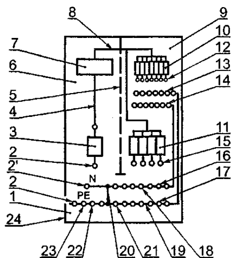
Рисунок Б.3 — Схема расположения аппаратуры в однопанельном ВПУ
